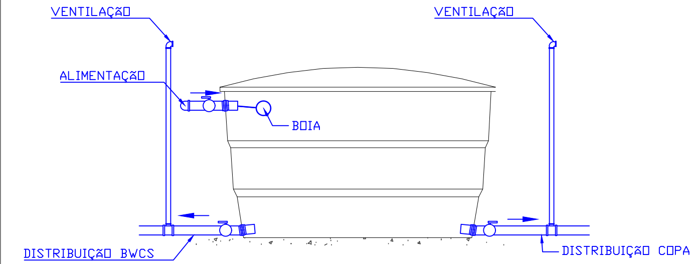
DETALHAMENTO CAIXA D'ÁGUA S/ Esc
