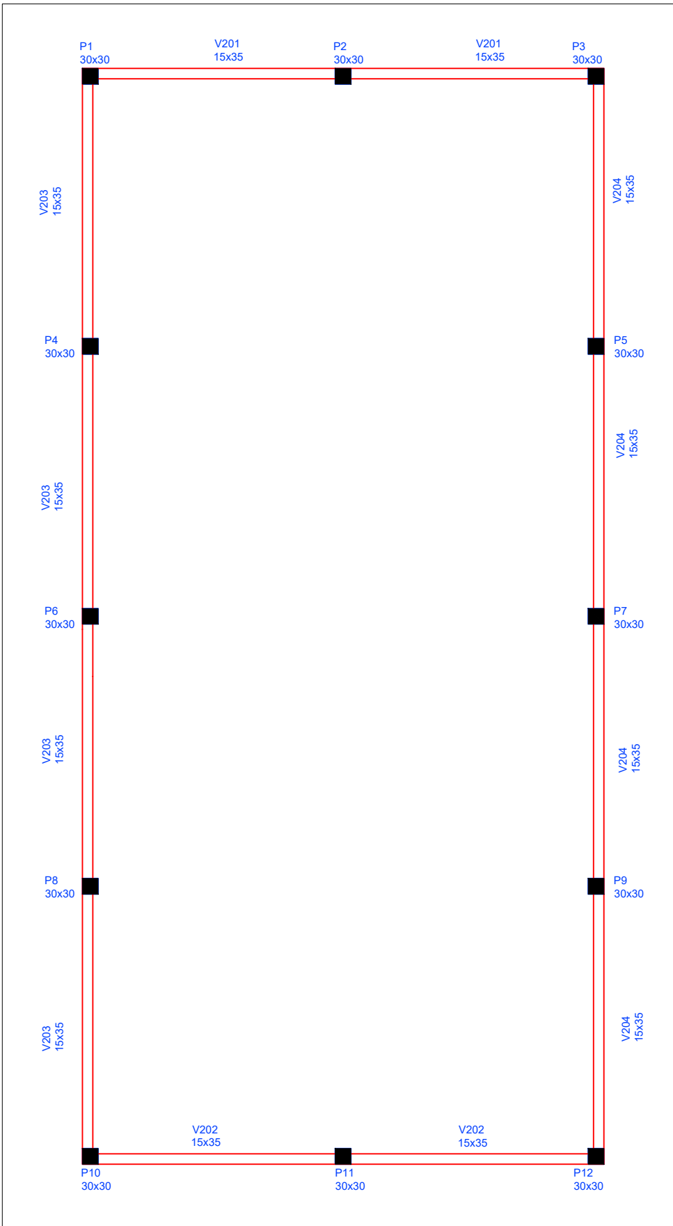
VIGAS SUPERIORES Esc= 1:100
