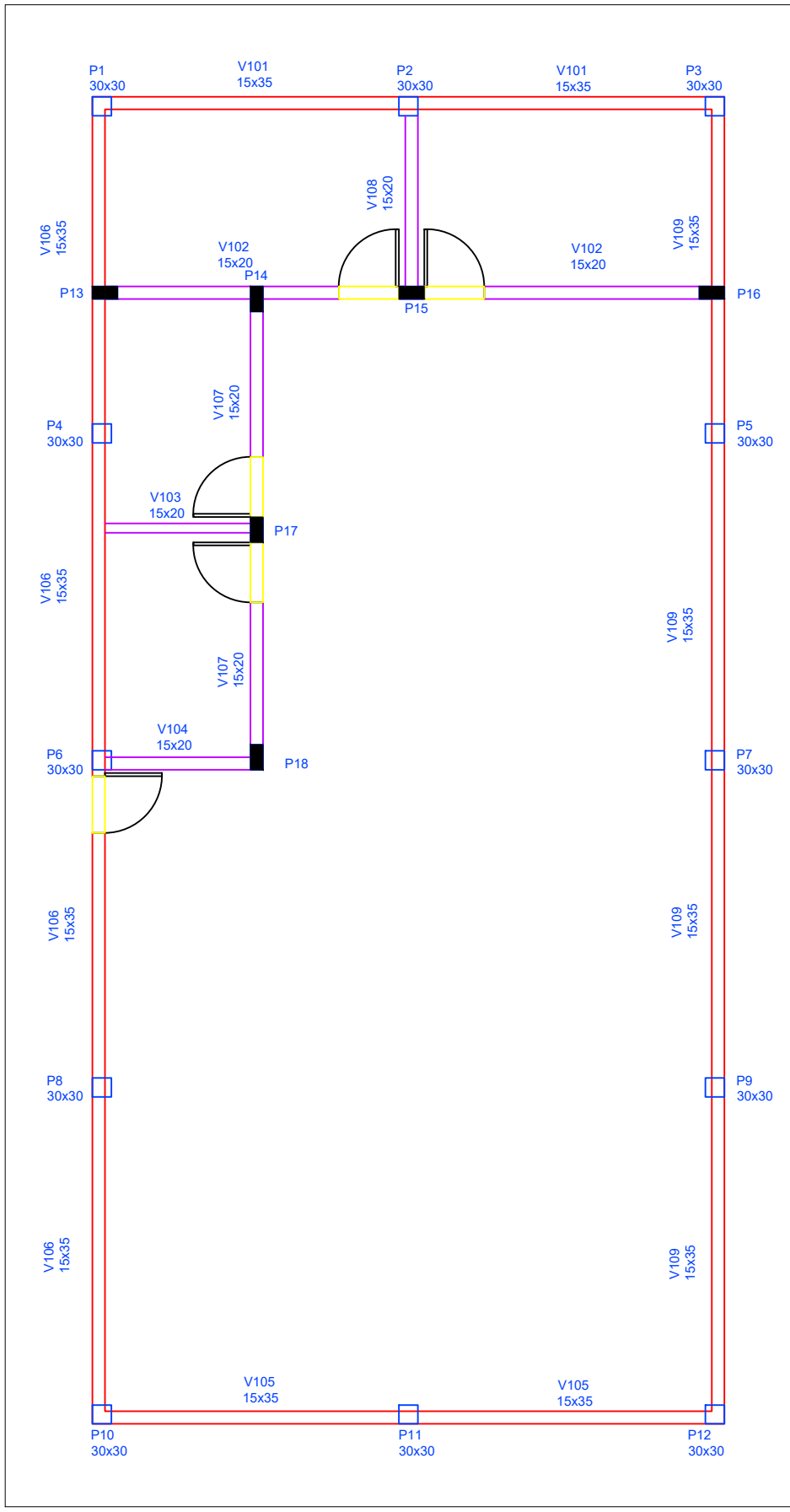
VIGAS INTERMEDIÁRIAS Esc= 1:100
