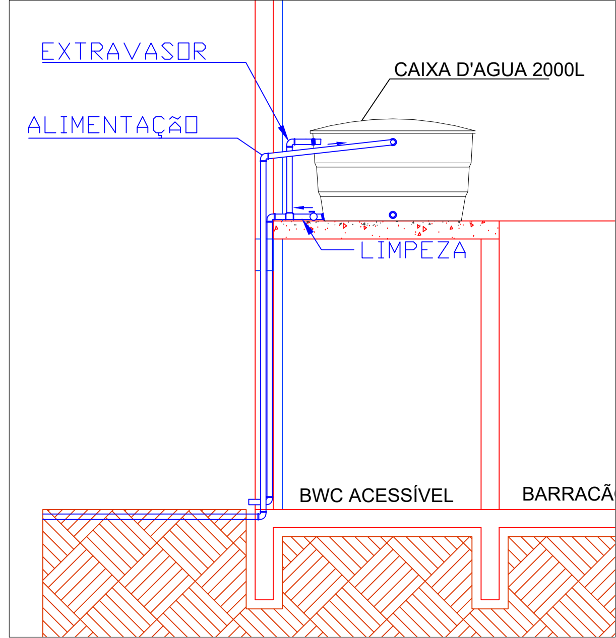
DETALHAMENTO CAIXA D'ÁGUA S/ Esc
