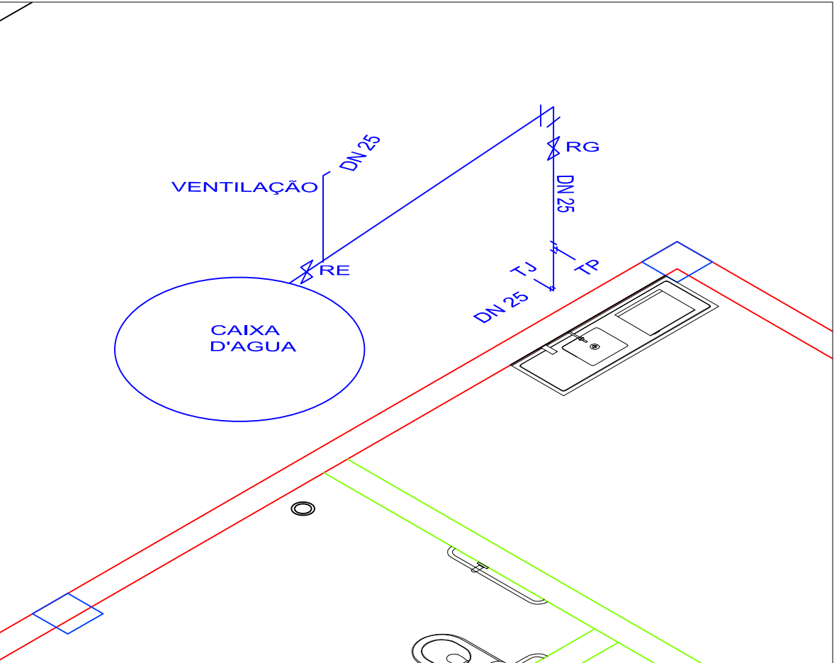
ISOMÉTRICO COPA S/ Esc
