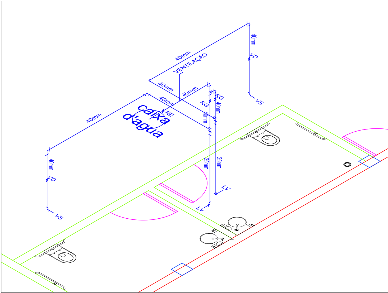
ISOMÉTRICO BWCs S/ Esc
