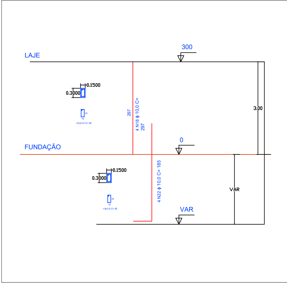
VIGAS INTERMEDIÁRIAS Esc= 1:100
